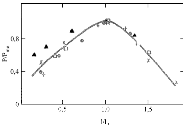
Рис. 1. Зависимость экспериментальных значений амплитуды давления от длины МЭП при: \square – C = 0,56 мкФ, U_0 = 40 кВ; + - C = 0,56 мкФ, U_0 = 60 кВ; \bullet – C = 0,56 мкФ, U_0 = 80 кВ; \blacktriangle – C = 0,56 мкФ, U_0 = 42,5 кВ; \times – C = 3 мкФ, U_0 = 40 кВ; L = 3 мкГн; сплошная линия – результат осреднения всех опытных данных [10].
